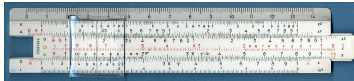
Slika 8.2 Drsko računalo. Osnovni skali sta D in drseči C. Računalo kaže produkt 1,24 \cdot 1,32 = 1,64 . Hkrati kaže kvocient 1,64/1,32 = 1,24 . Skala A je kvadrat skale D in kaže 1,64^2 = 2,7 oziroma \sqrt{2,7} = 1,64 . Podobno velja za skalo K, ki je kub skale D. Skala L pa je logaritem skale D in kaže \lg 1,64 = 0,215 . (Anon)
