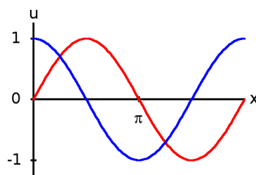
Slika 10.6 Graf sinusne funkcije u = \sin x (rdeča črta) in kosinusne funkcije u = \cos x (modra črta). Prikazana je le osnovna perioda vsake funkcije. Ta perioda se ponavlja v levo in v desno brez konca.
