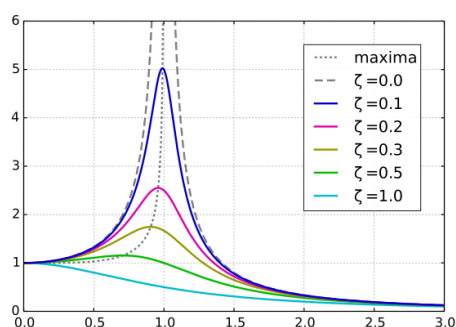
Slika 18.1 Resonantna krivulja pri različnih dušenjih. Na abscisi je razmerje \omega/\omega_0 in na ordinati ojačanje amplitude R . (Anon.)
