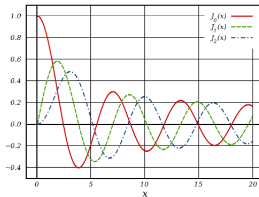
Slika 18.3 Cilindrične funkcije kot rešitve amplitudne enačbe v cilindričnih koordinatah. (Anon)
