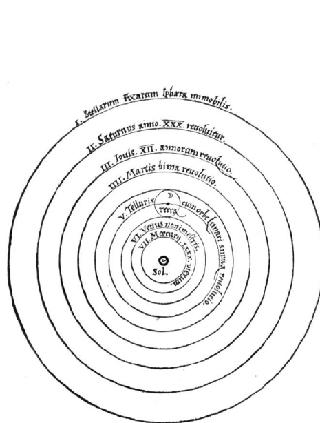
Slika 7.15 Heliocentrični sistem sveta. Sonce je v središču, okrog njega krožijo planeti. Luna kroži okoli Zemlje. (Kopernik, 1543)
