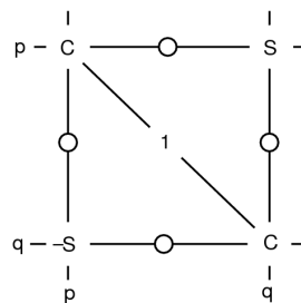
Slika 14.7 Diagonalizacija matrike s primernim vrtenjem.
